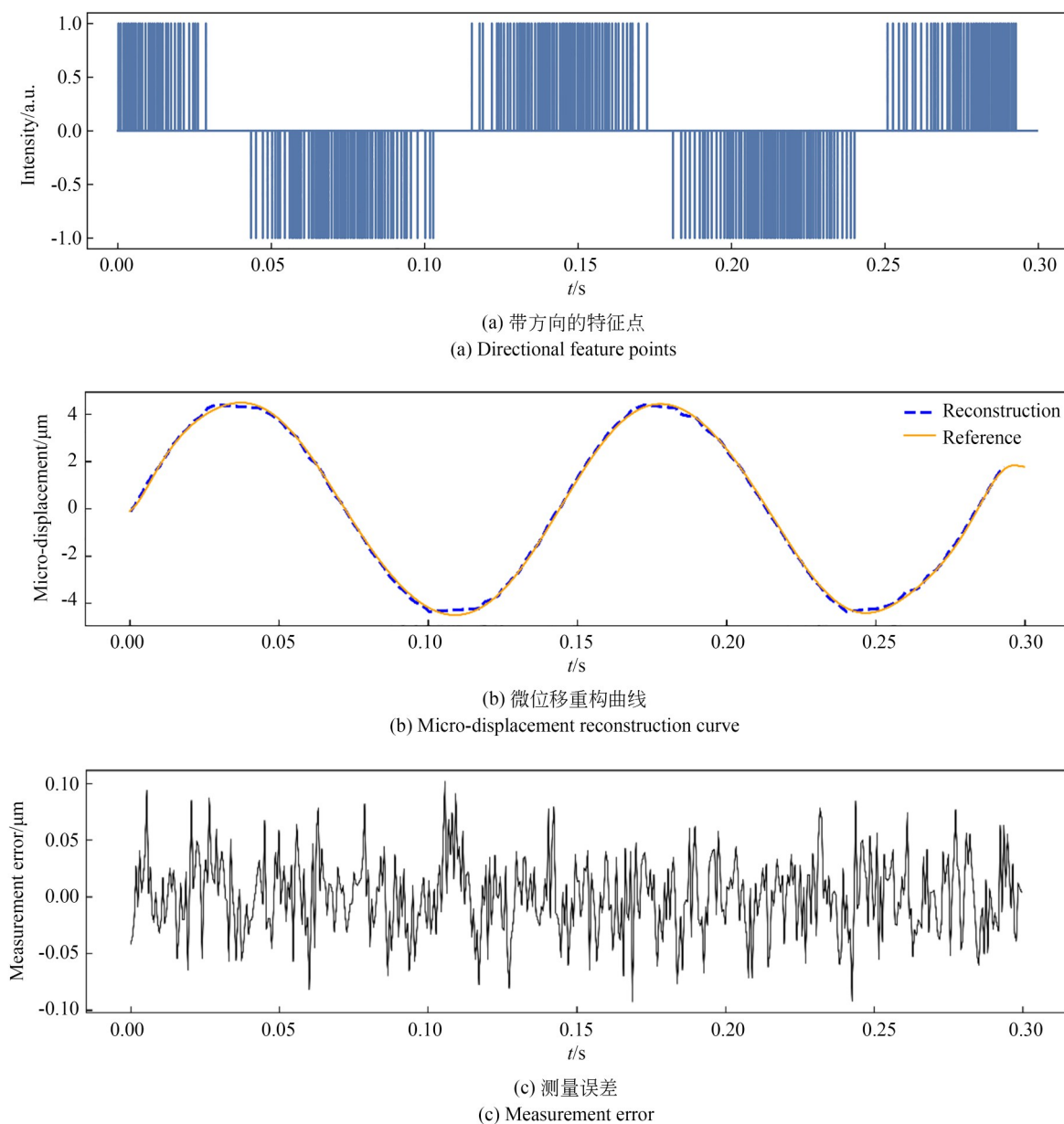
图 5 双波长单纵模掺镱光纤激光器自混合干涉微位移测量实验数据处理及结果
